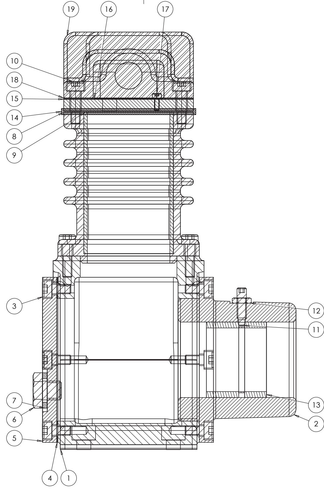
COUPE A-A ECHELLE 3:2
