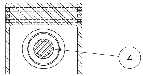
COUPE B-B
