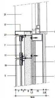
COUPE HORIZONTALE
